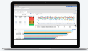
Top N
